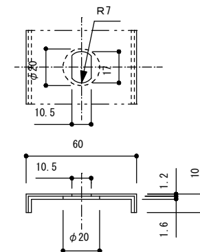
フック用穴部詳細 (S=1/2)
