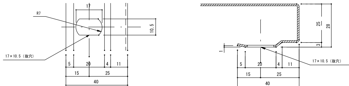
A部断面詳細 (S= 1 / 1)
