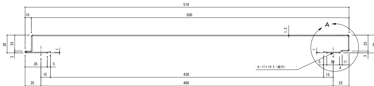
断面詳細図 (S= 1 / 2)
