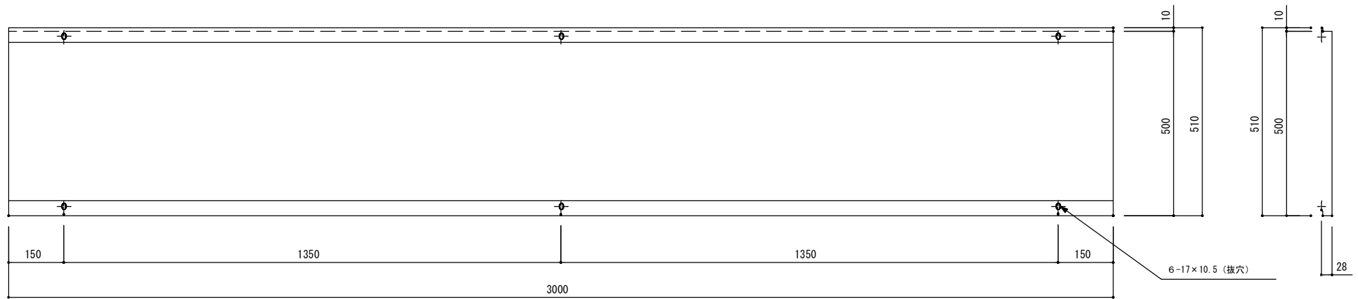
断面詳細図 (S= 1 / 2)
