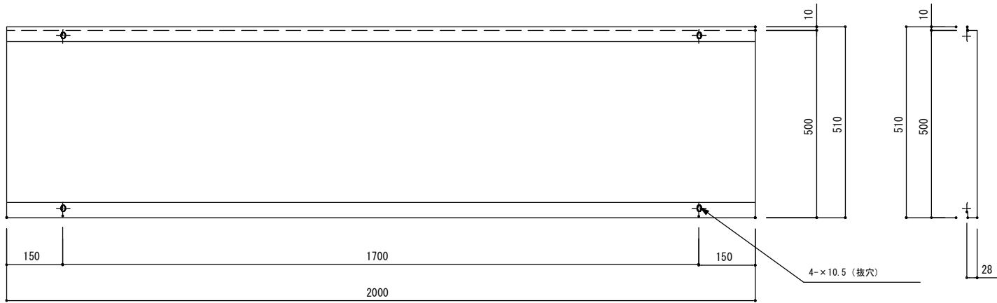
断面詳細図 (S=1/2)
